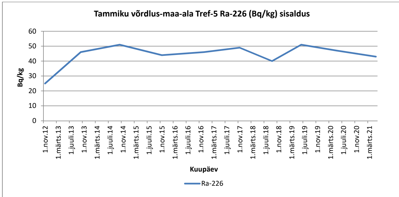
Graafik 94. Ra-226
