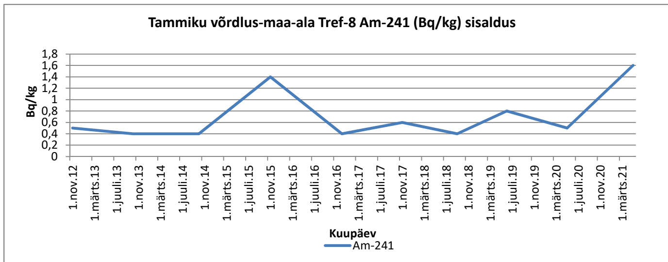
Graafik 111. Am-241
