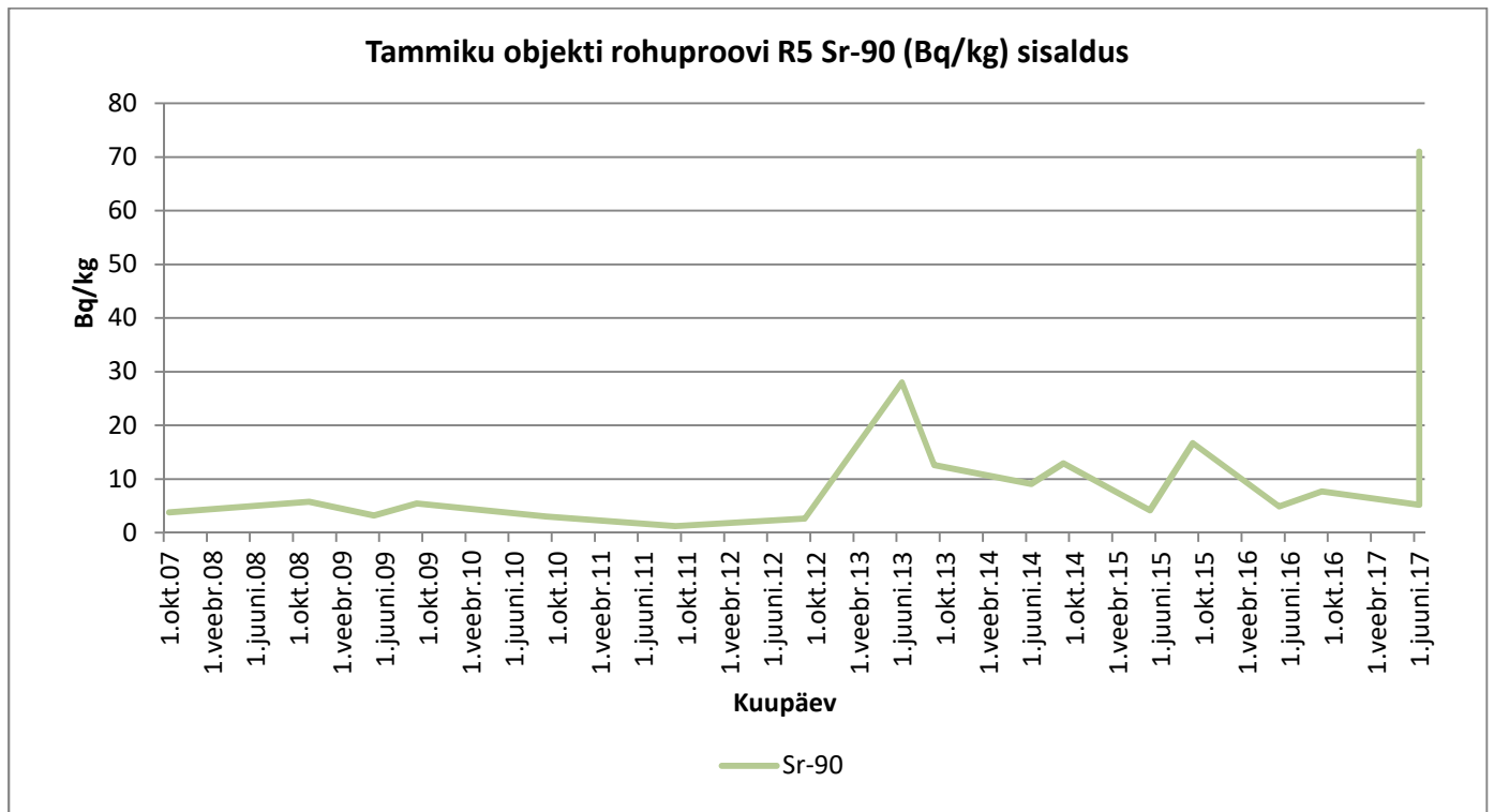
Graafik 14. Sr-90
