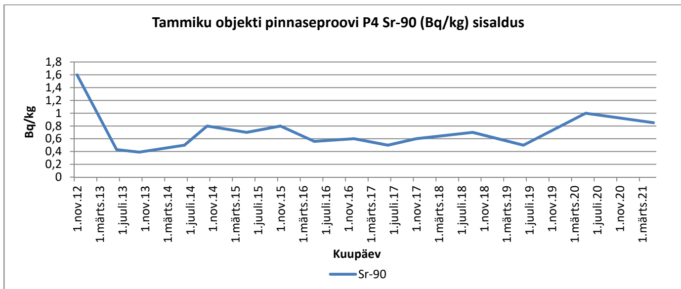
Graafik 47. Sr-90
