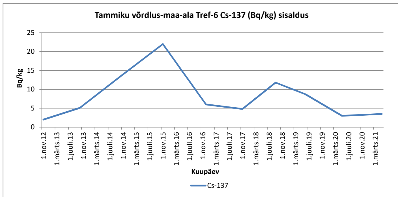
Graafik 97. Cs-137
