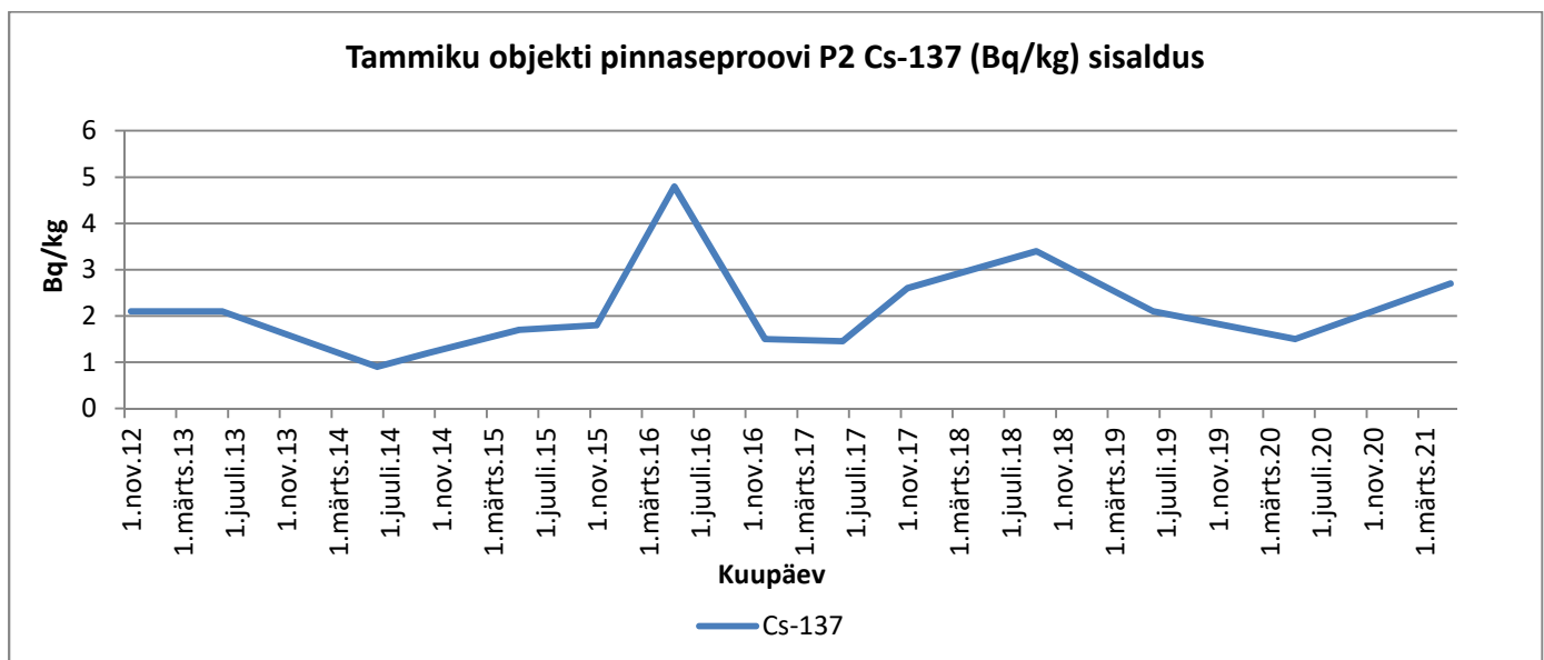
Graafik 39. Cs-137
