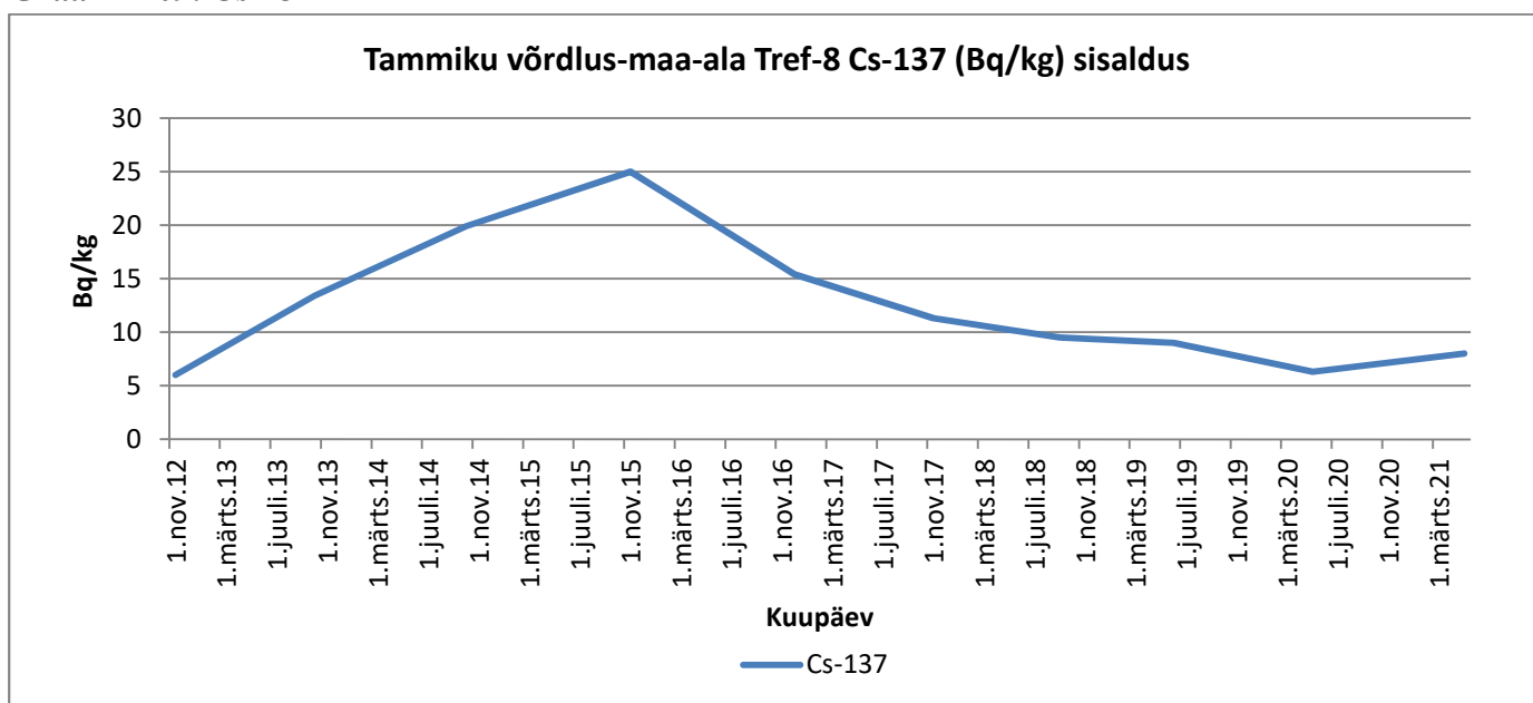
Graafik 109. Cs-137
