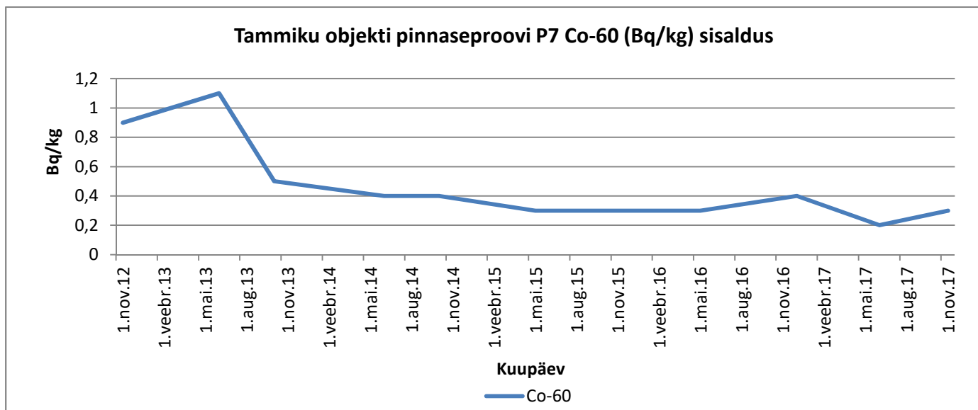
Graafik 61. Co-60
