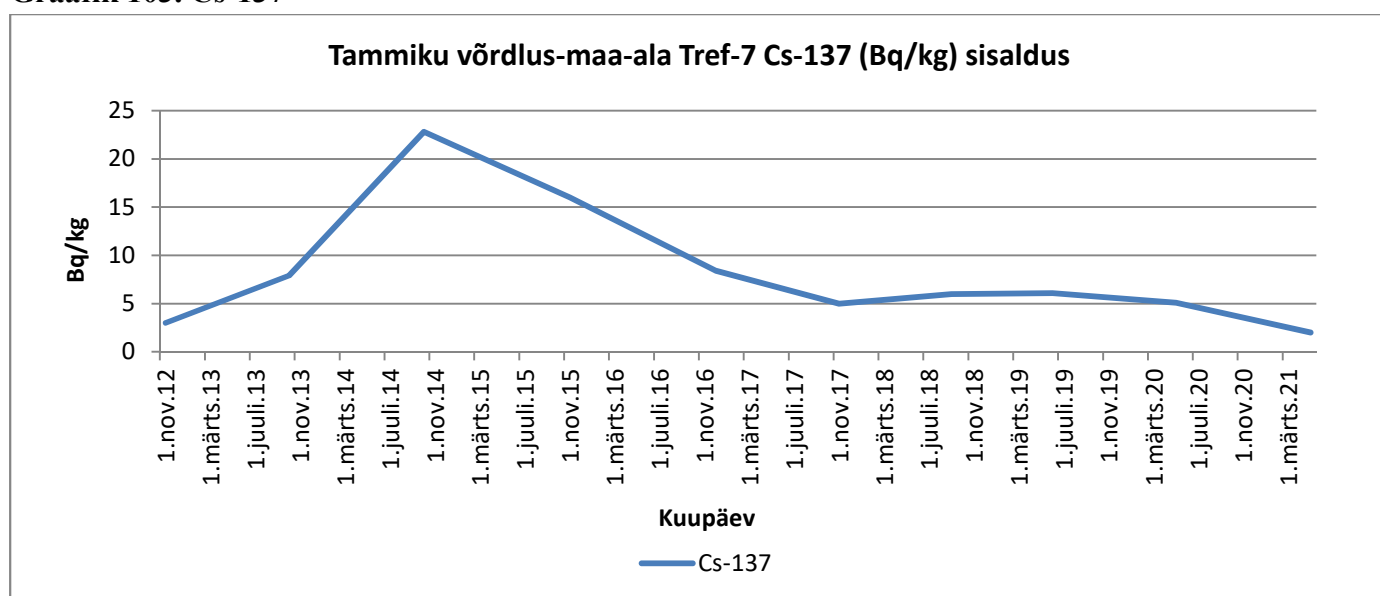
Graafik 103. Cs-137
