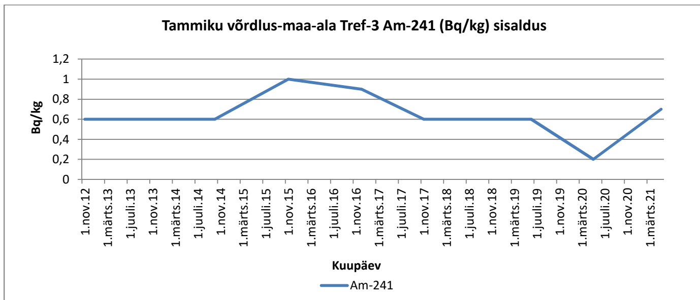
Graafik 81. Am-241
