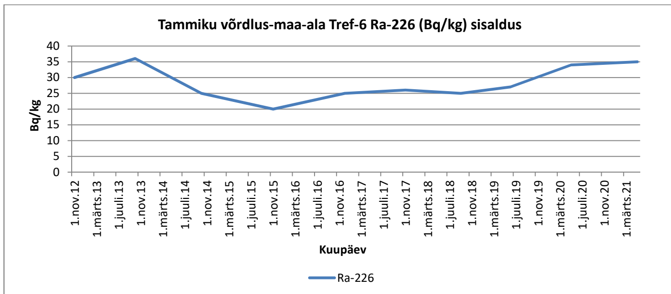
Graafik 100. Ra-226
