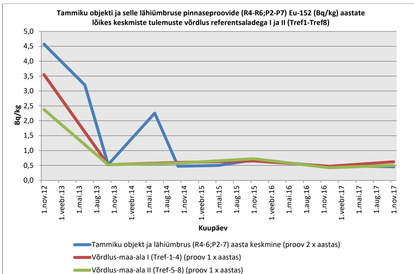
Graafik 118. Eu-152
