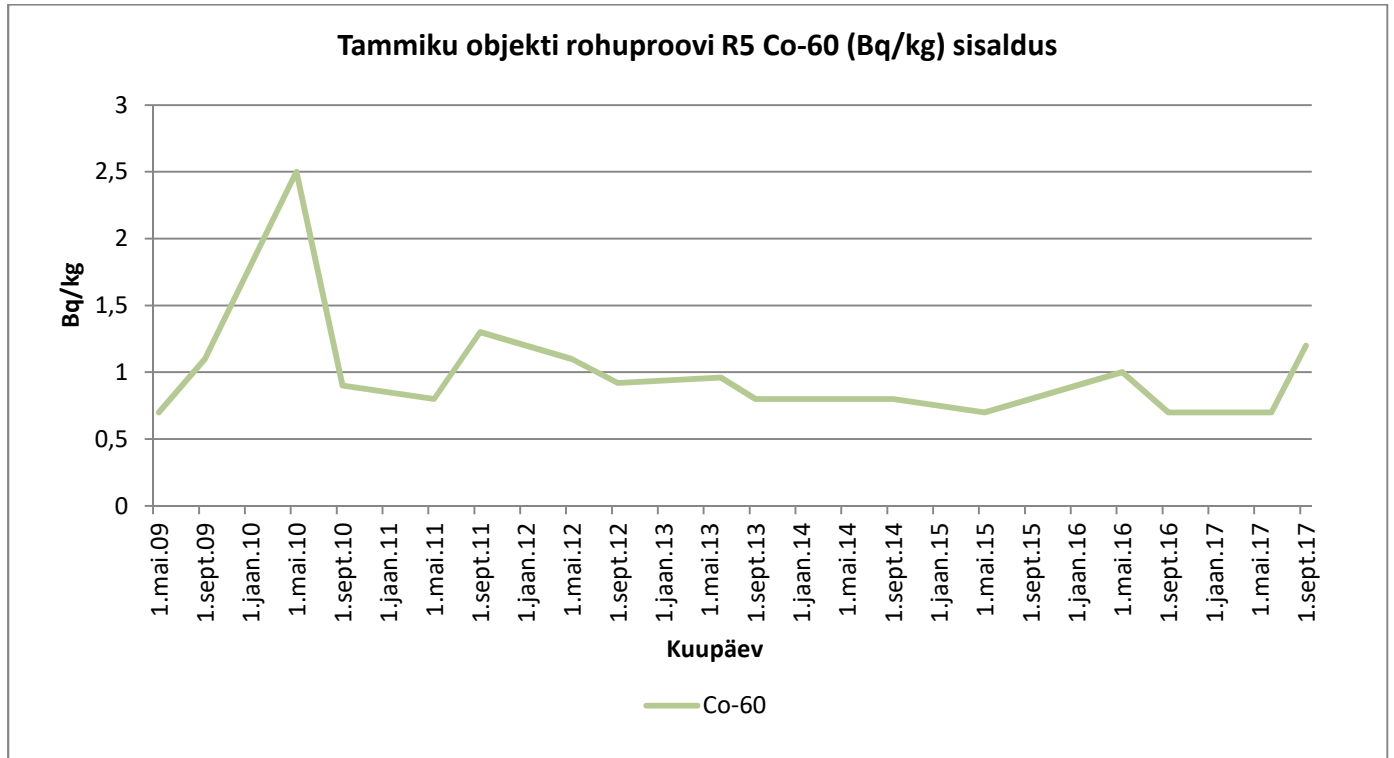
Graafik 13. Co-60
