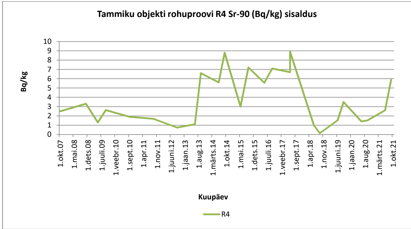
Graafik 11. Sr-90
