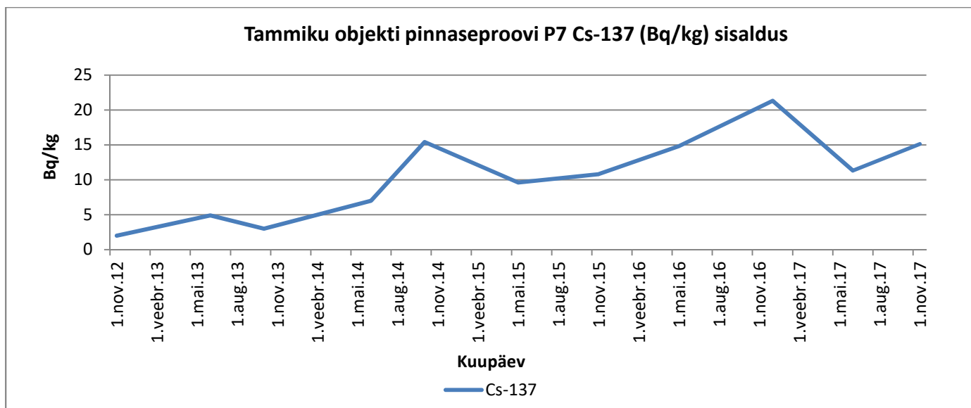
Graafik 60. Cs-137
