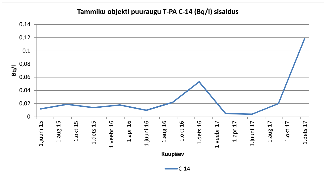
Graafik 8. C-14
