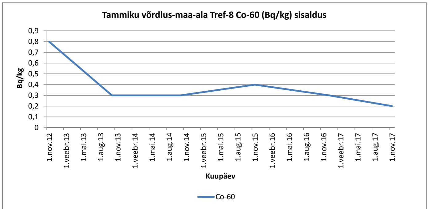
Graafik 114. Co-60
