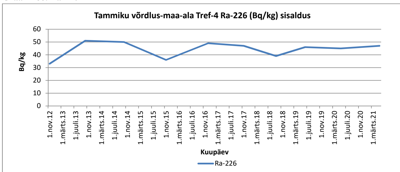
Graafik 88. Ra-226
