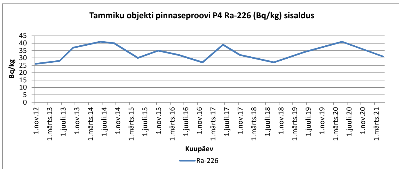
Graafik 49. Ra-226
