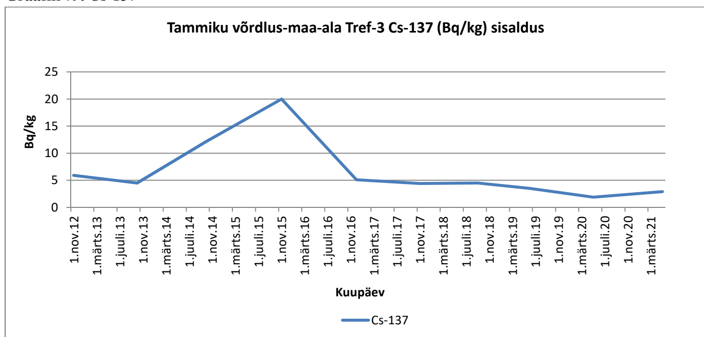
Graafik 79. Cs-137
