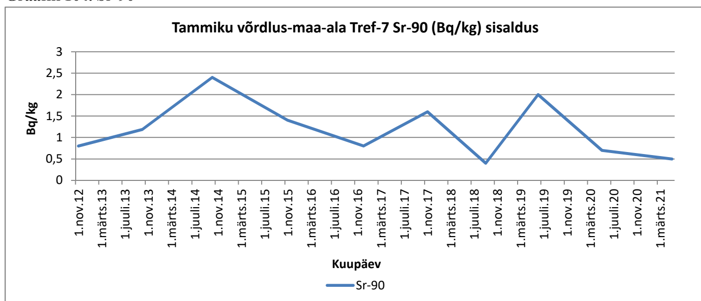
Graafik 104. Sr-90
