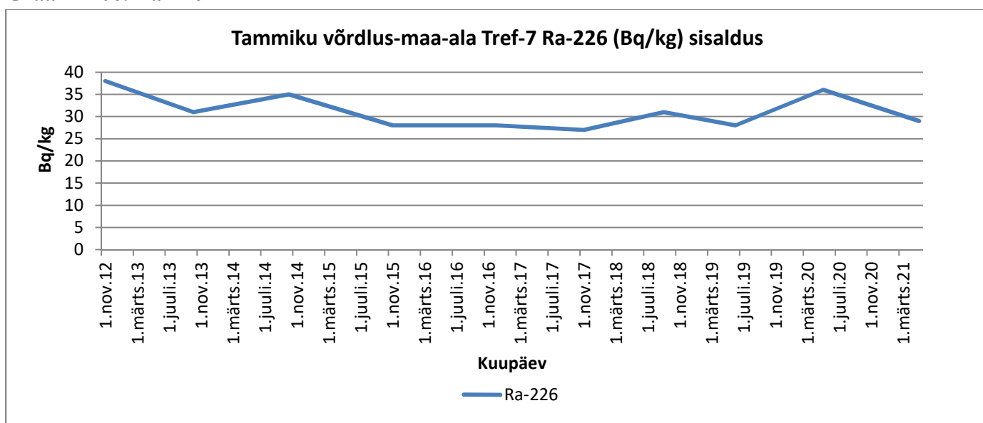
Graafik 106. Ra-226
