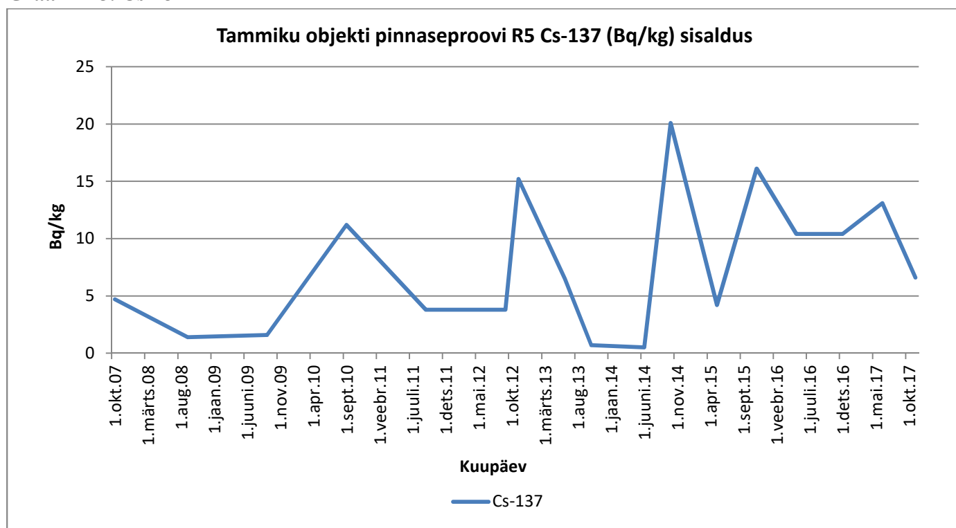
Graafik 25. Cs-137
