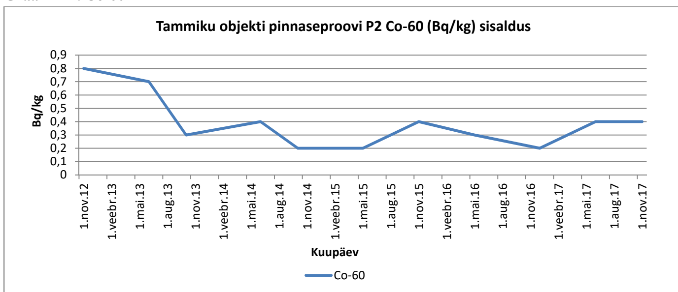
Graafik 44. Co-60
