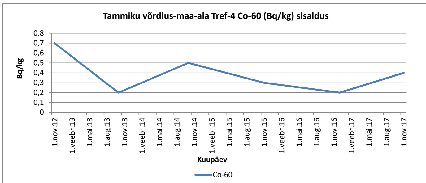
Graafik 90. Co-60
