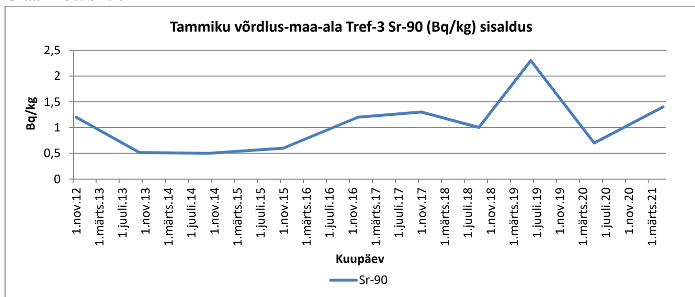
Graafik 80. Sr-90
