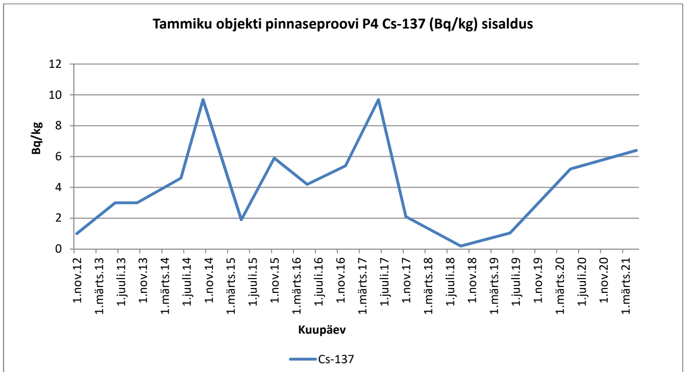
Graafik 46. Cs-137
