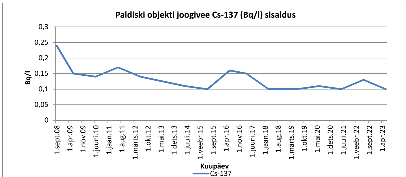
Graafik 14. Cs-137
