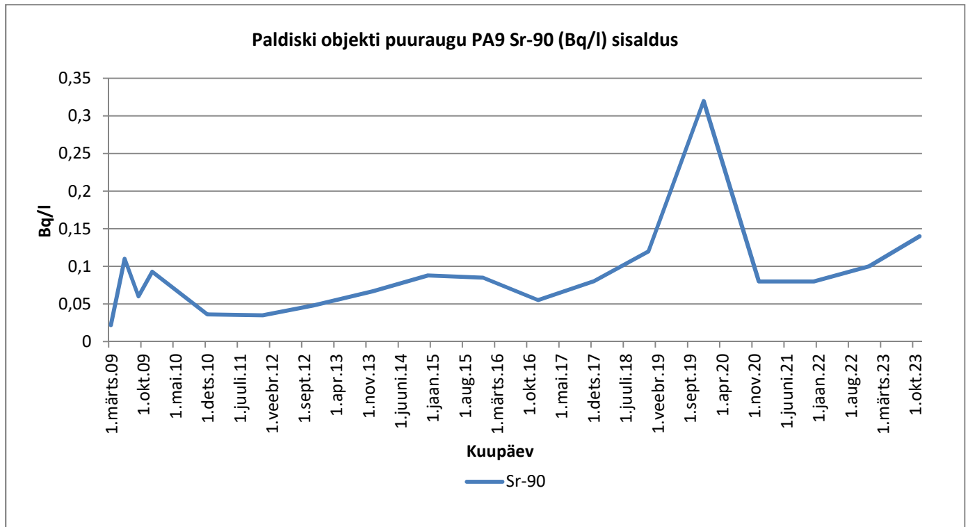
Graafik 12. Sr-90
