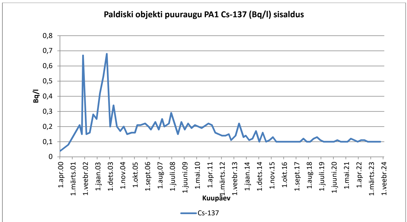
Graafik 2. Cs-137
