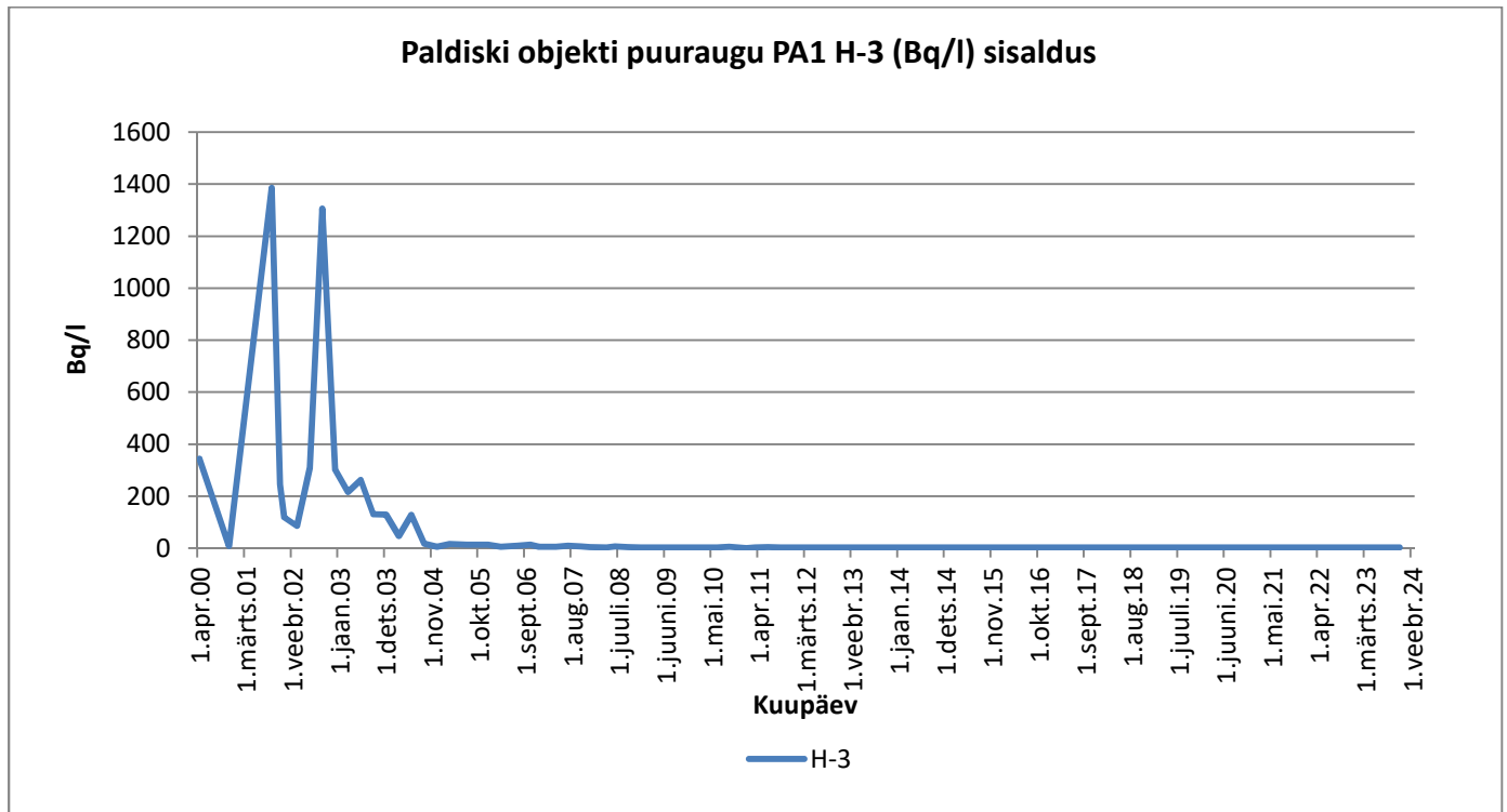
Graafik 1. H-3
