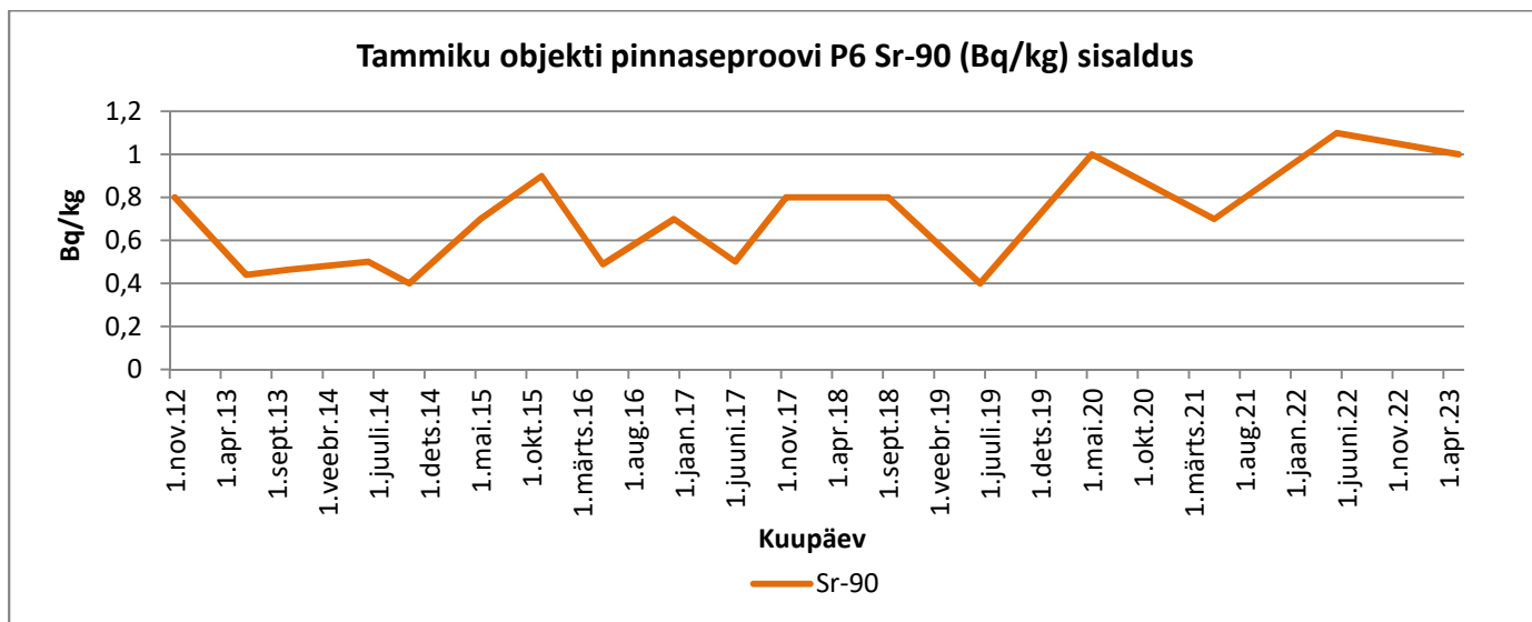
Graafik 54. Sr-90
