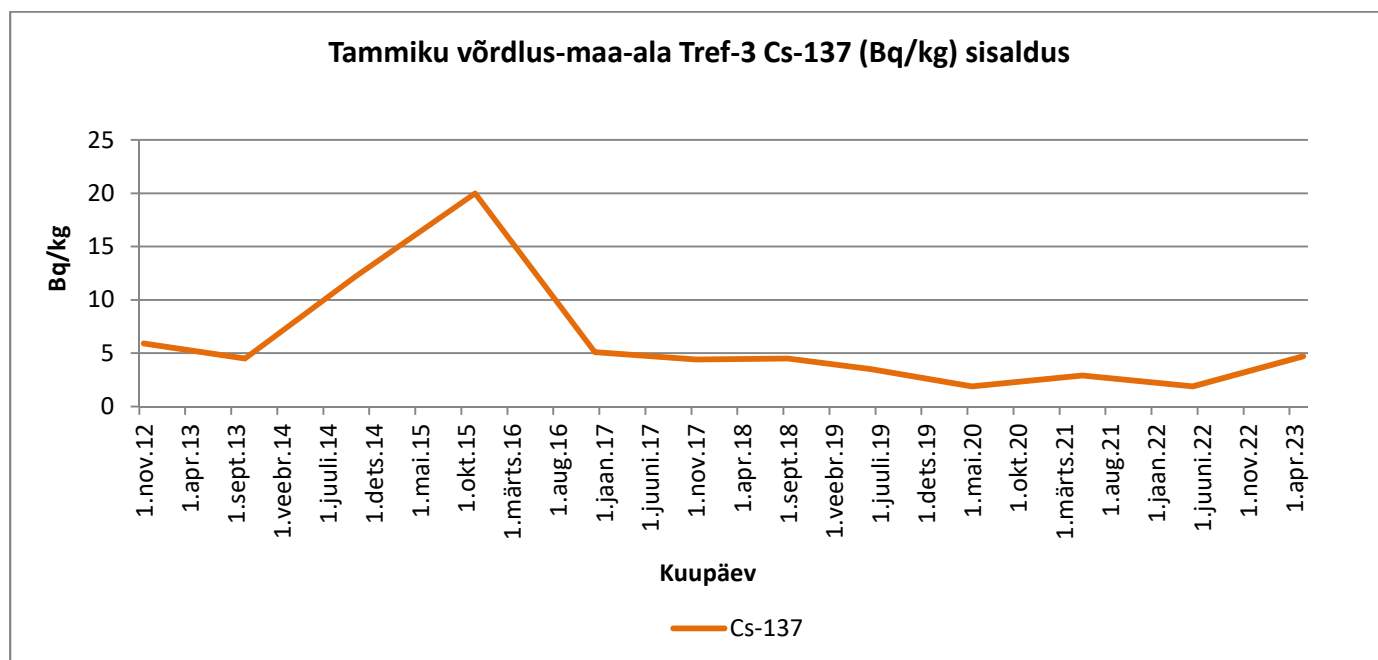
Graafik 79. Cs-137
