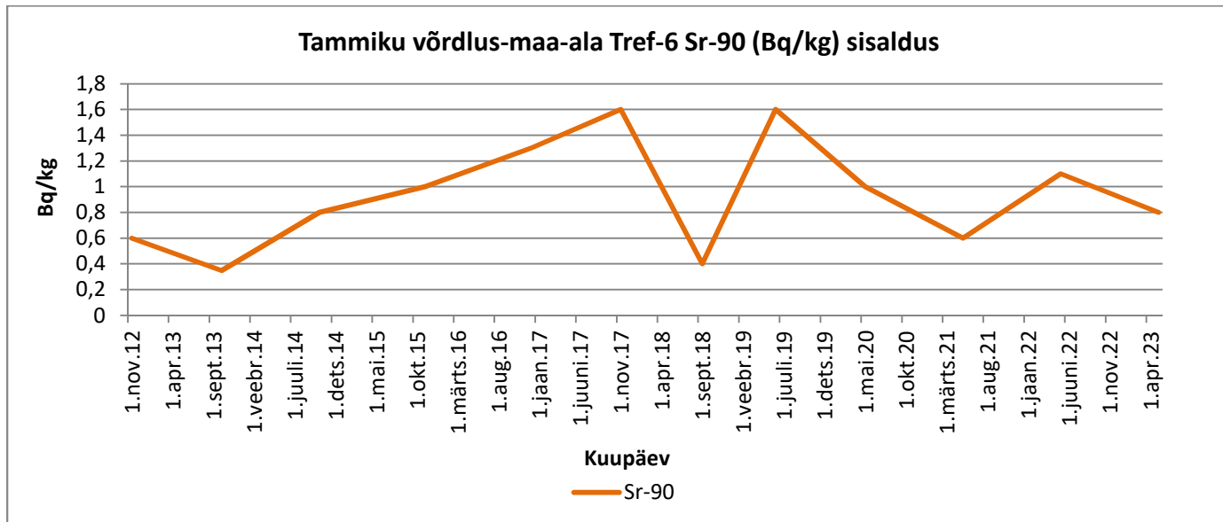
Graafik 98. Sr-90
