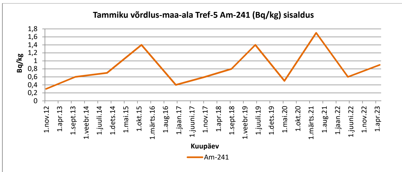
Graafik 93. Am-241
