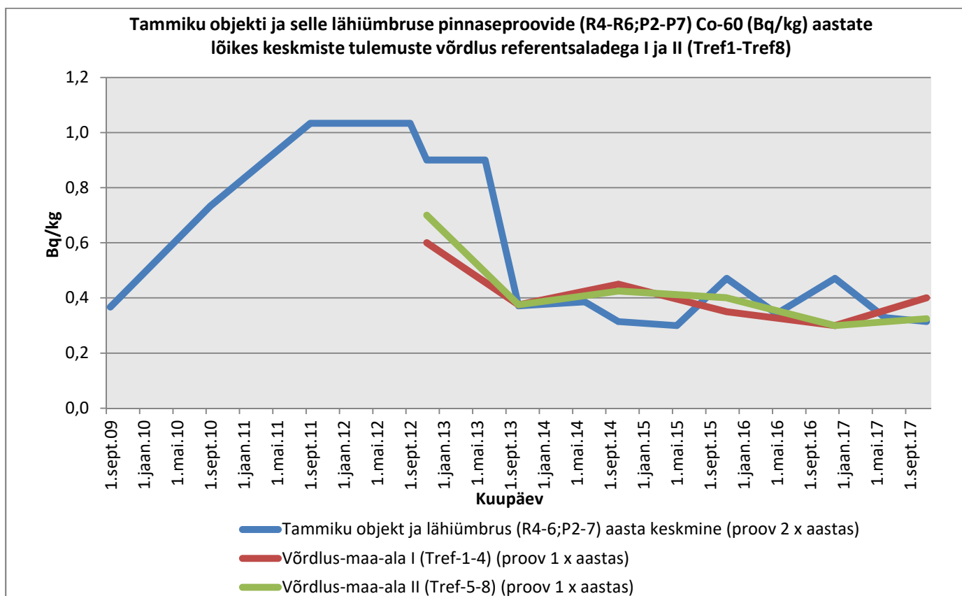
Graafik 116. Co-60
