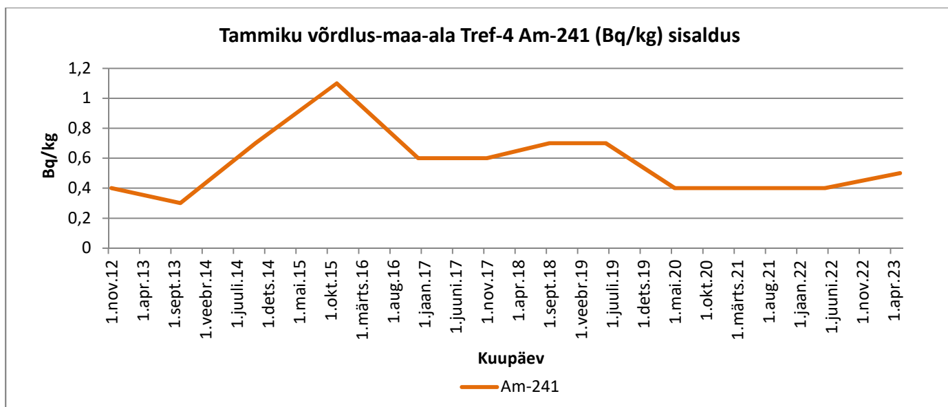
Graafik 87. Am-241
