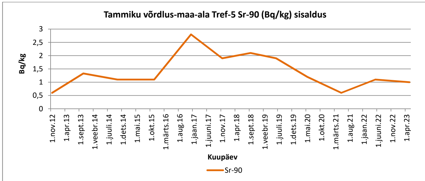
Graafik 92. Sr-90
