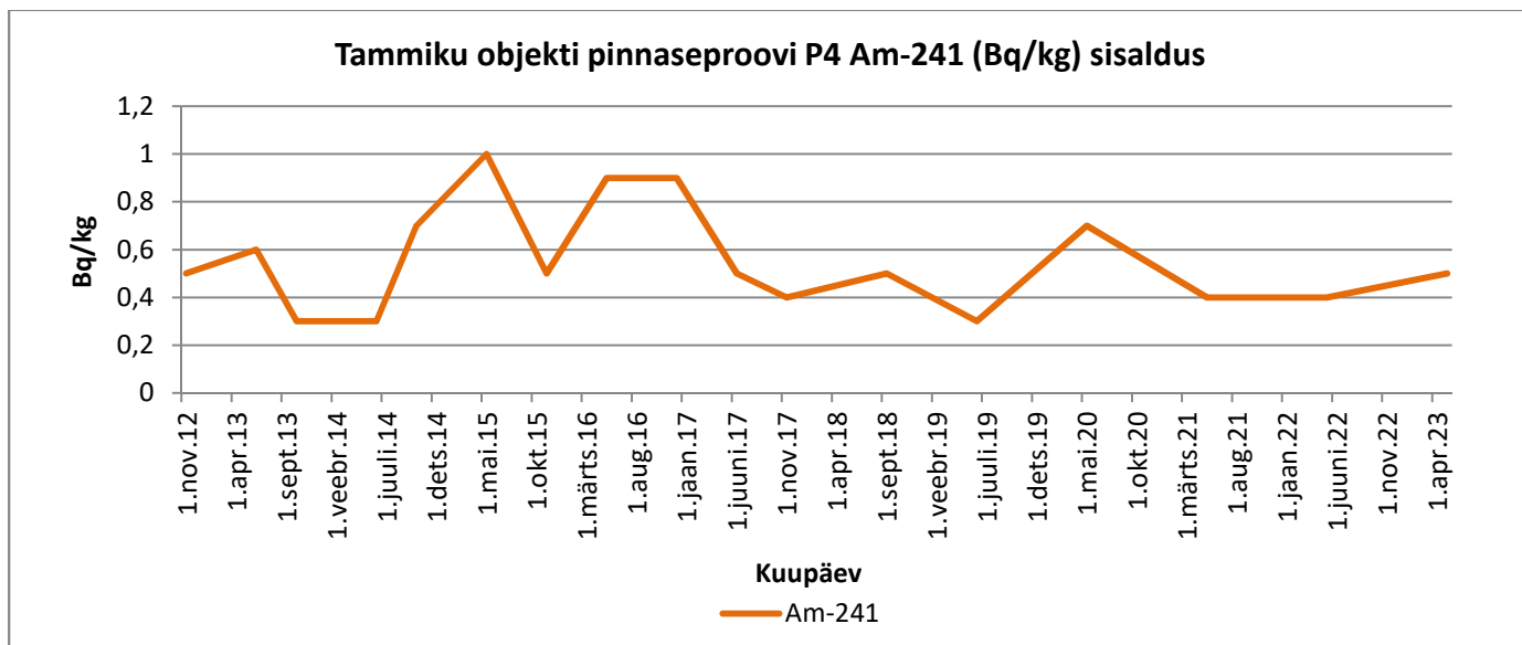
Graafik 48. Am-241
