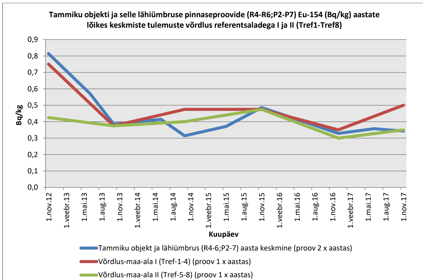
Graafik 119. Eu-154
