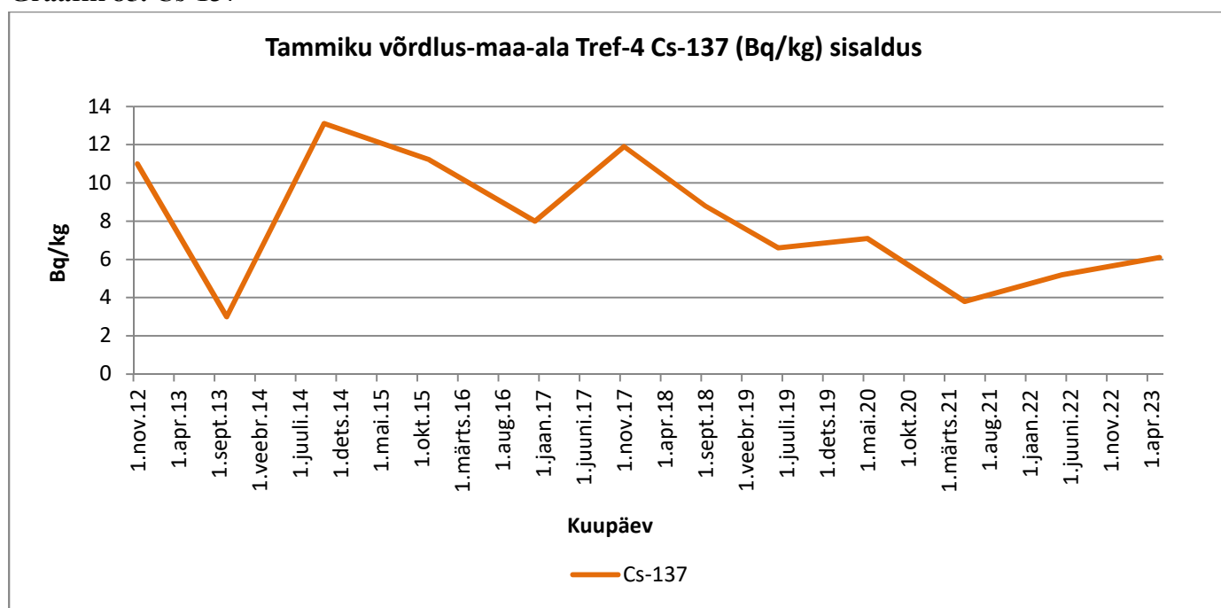
Graafik 85. Cs-137
