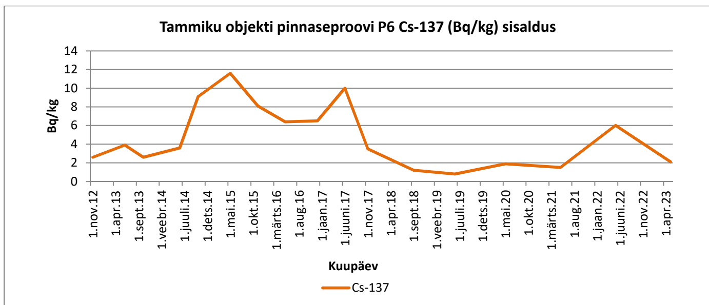
Graafik 53. Cs-137
