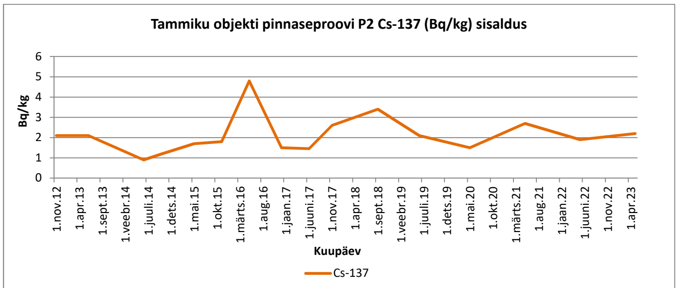
Graafik 39. Cs-137
