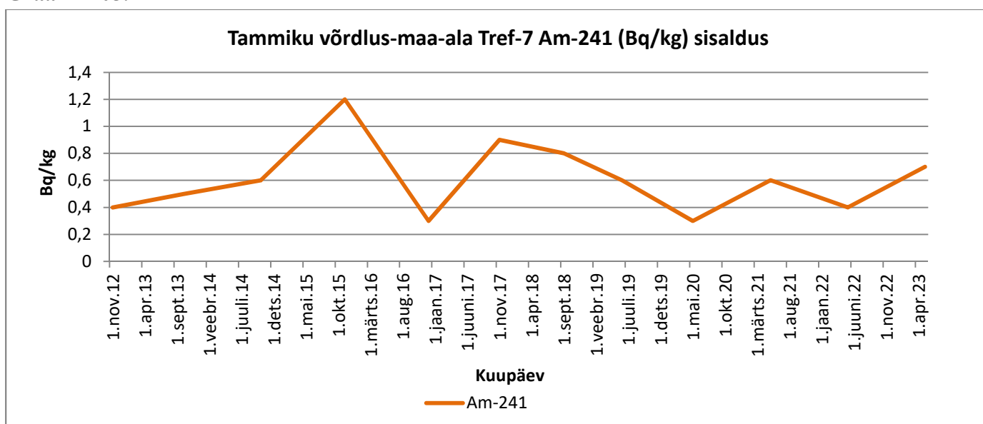
Graafik 105. Am-241
