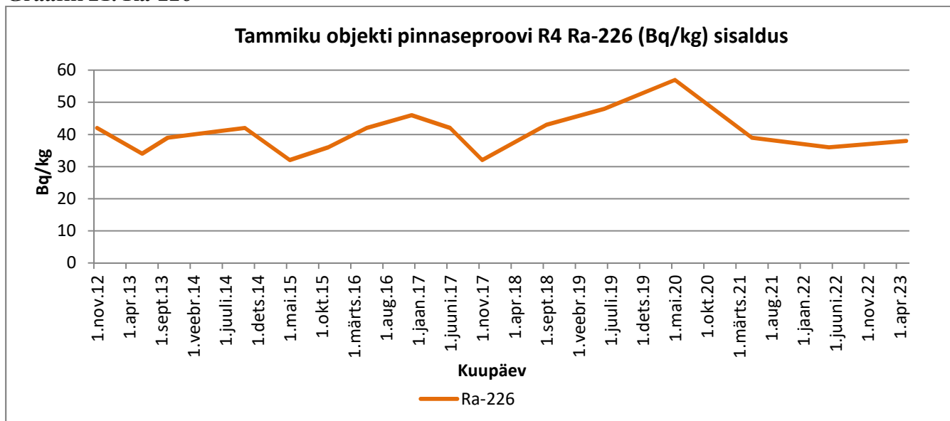
Graafik 21. Ra-226
