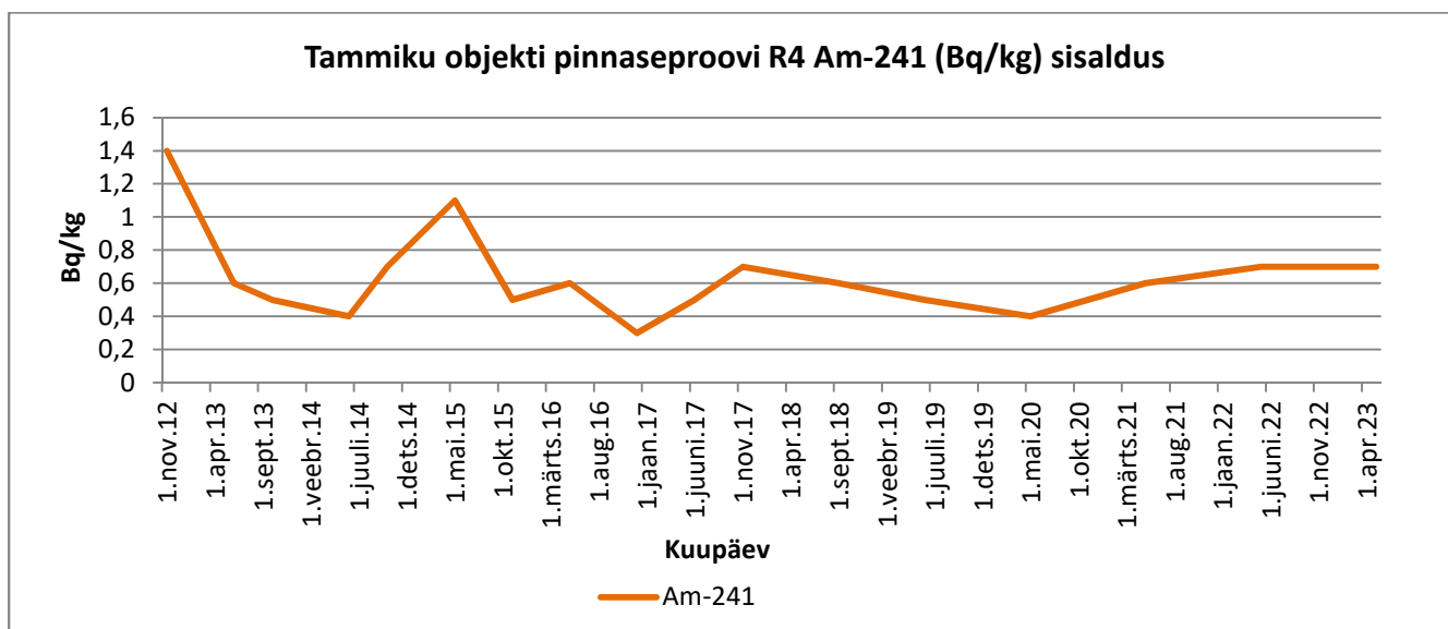
Graafik 20. Am-241
