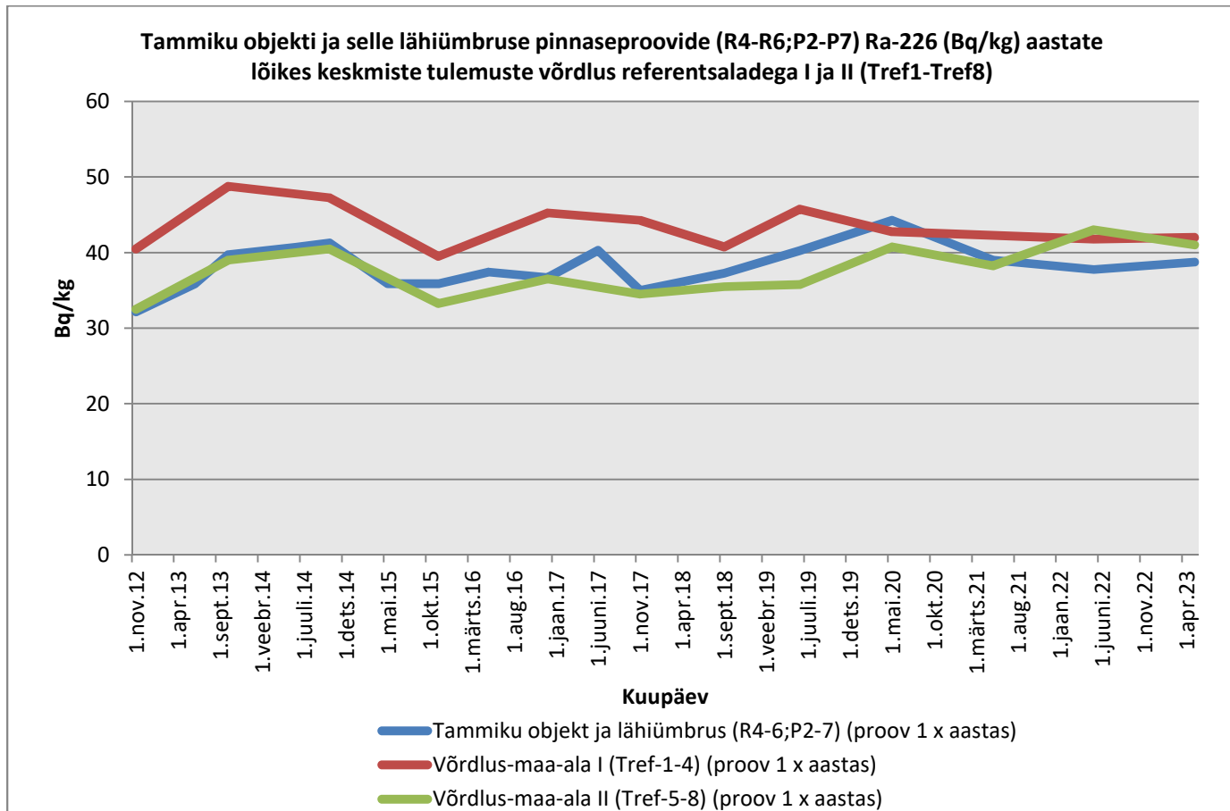
Graafik 121. Ra-226
