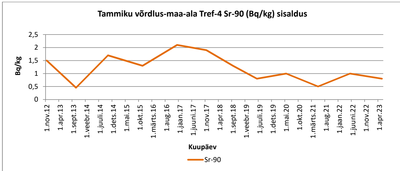
Graafik 86. Sr-90
