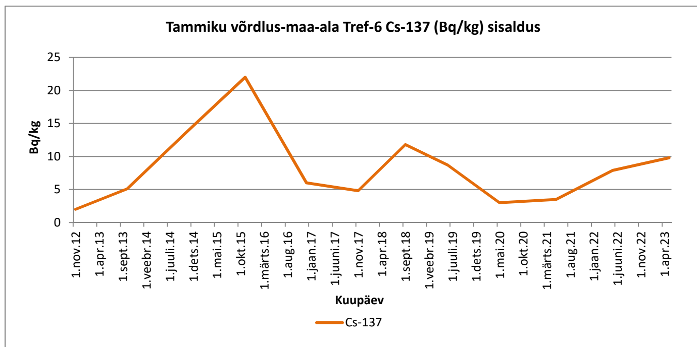
Graafik 97. Cs-137
