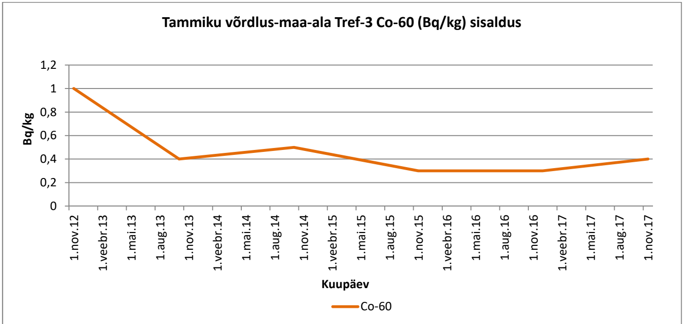
Graafik 84. Co-60
