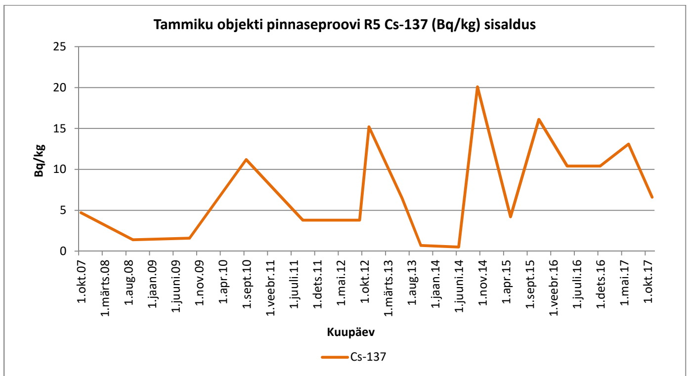
Graafik 25. Cs-137
