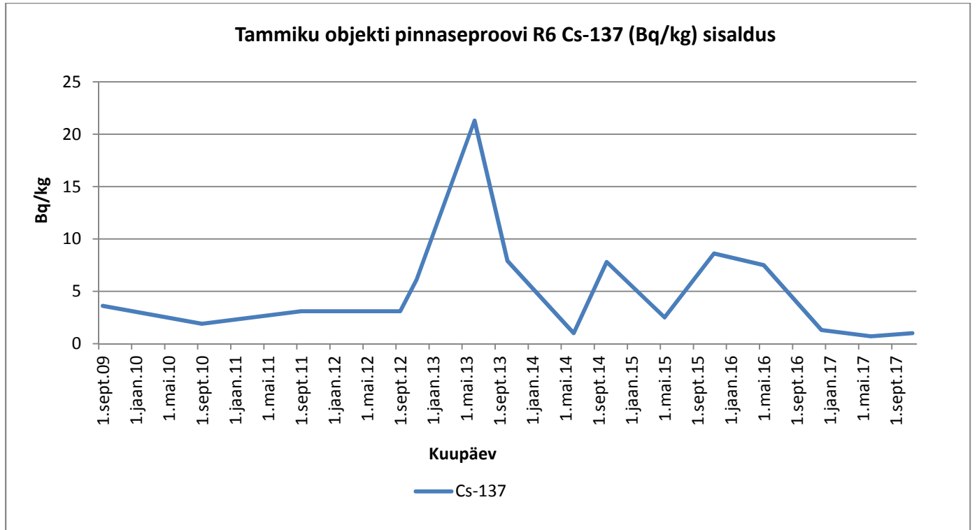
Graafik 32. Cs-137
