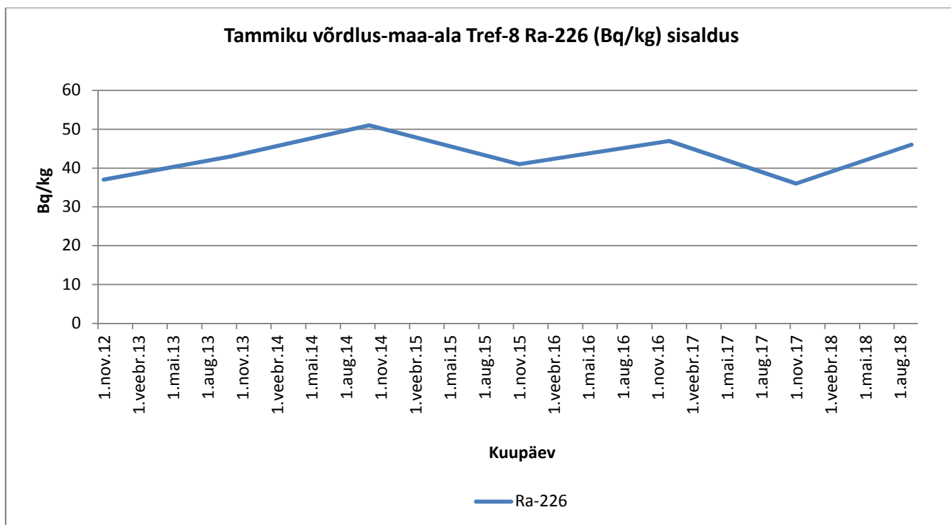
Graafik 112. Ra-226
