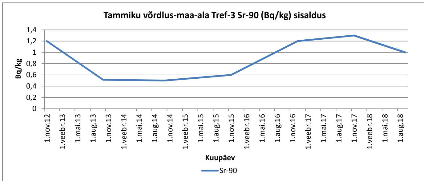
Graafik 80. Sr-90
