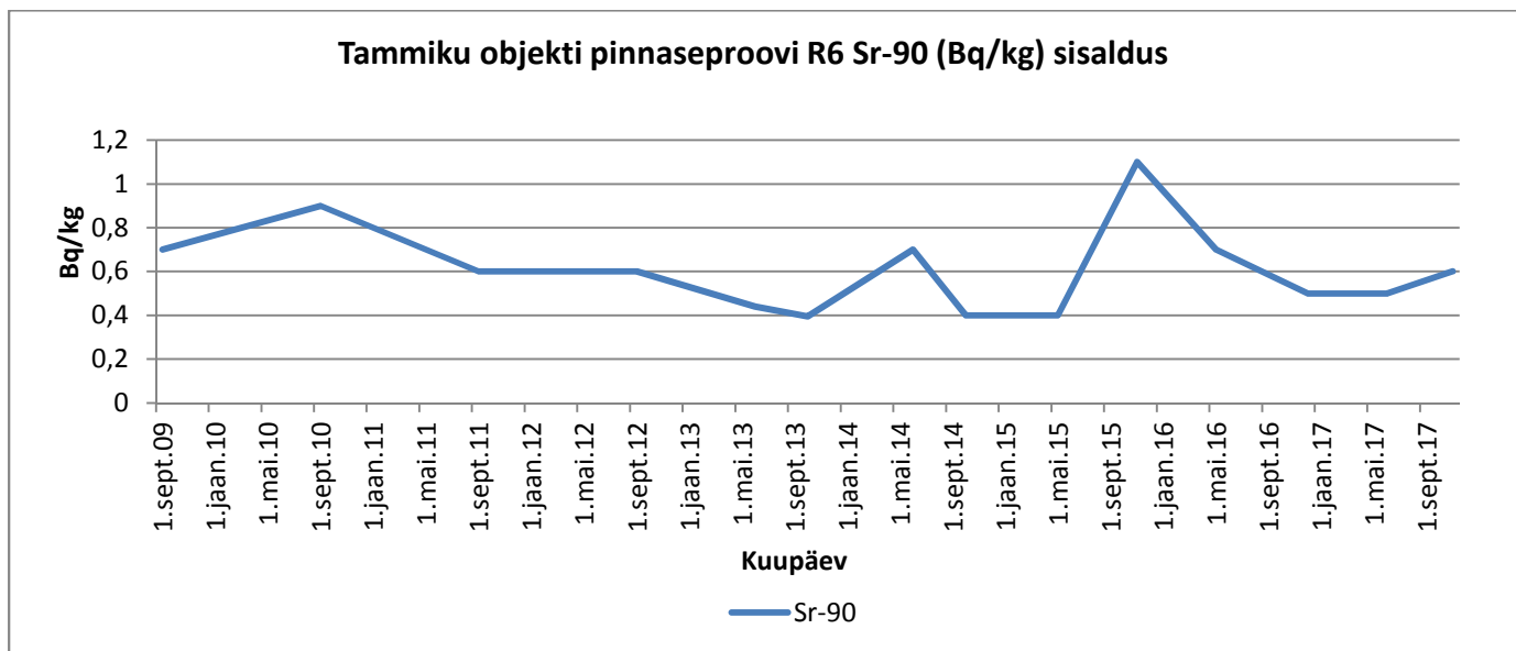
Graafik 34. Sr-90
