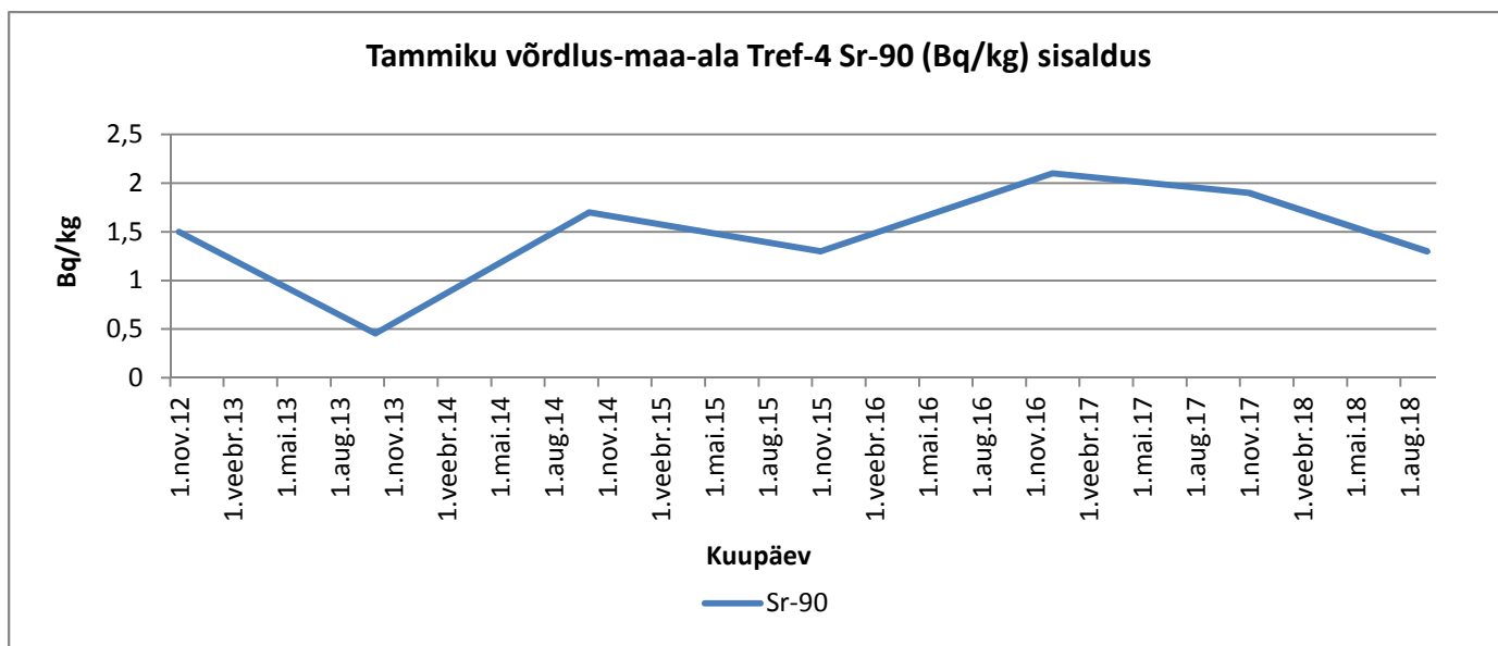
Graafik 86. Sr-90
