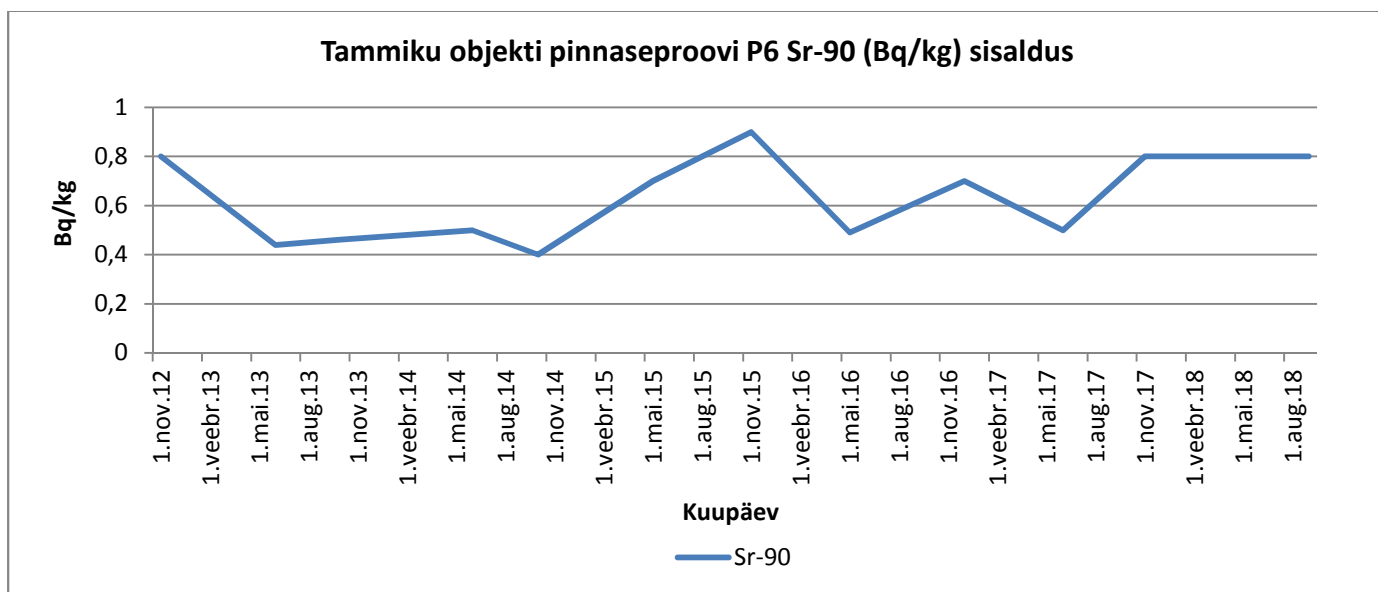
Graafik 54. Sr-90
