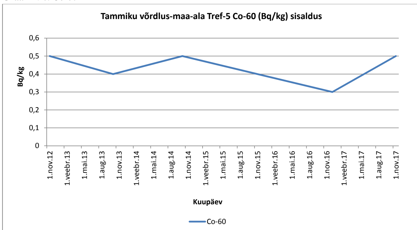
Graafik 96. Co-60
