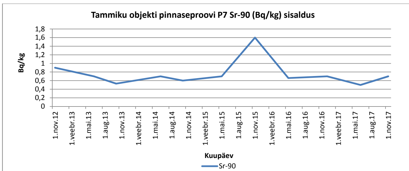
Graafik 62. Sr-90
