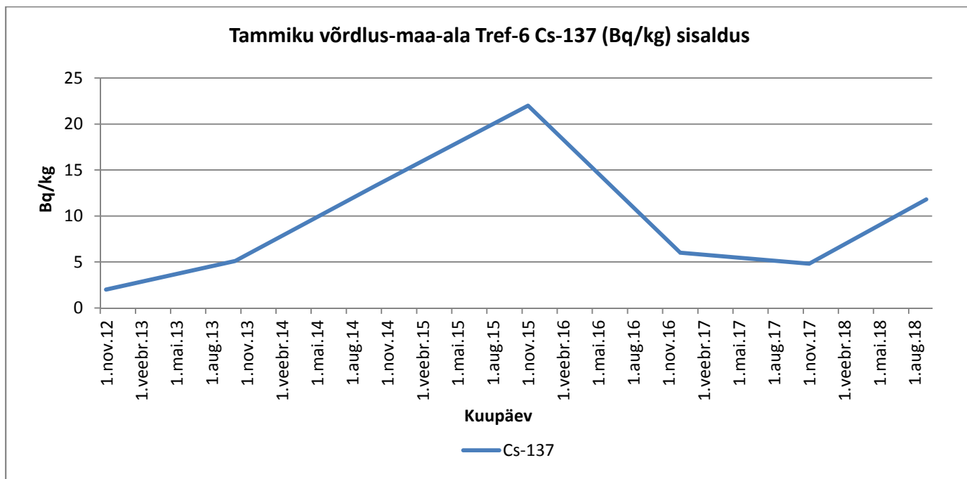
Graafik 97. Cs-137
