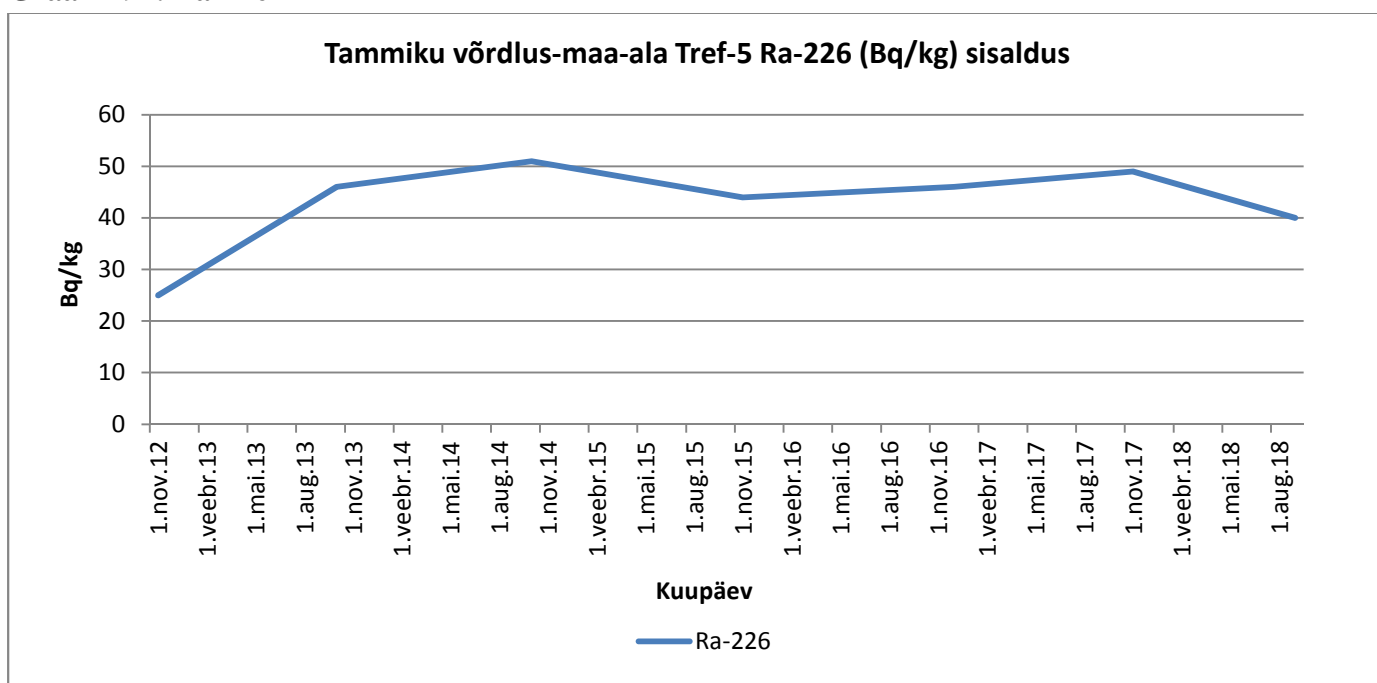
Graafik 94. Ra-226
