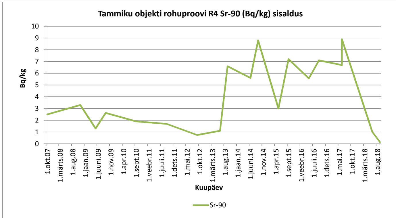
Graafik 11. Sr-90
