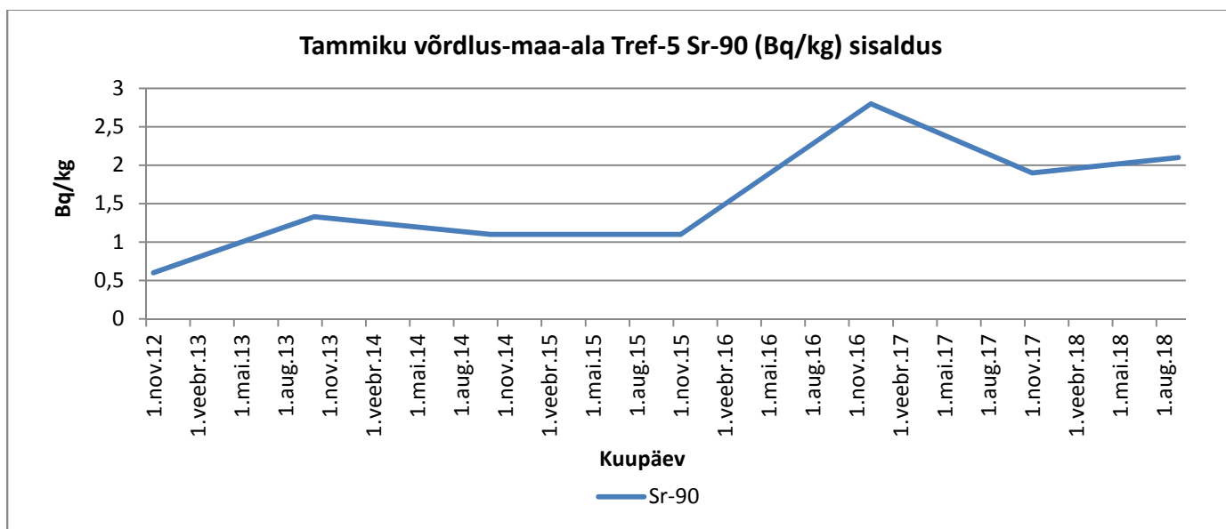
Graafik 92. Sr-90
