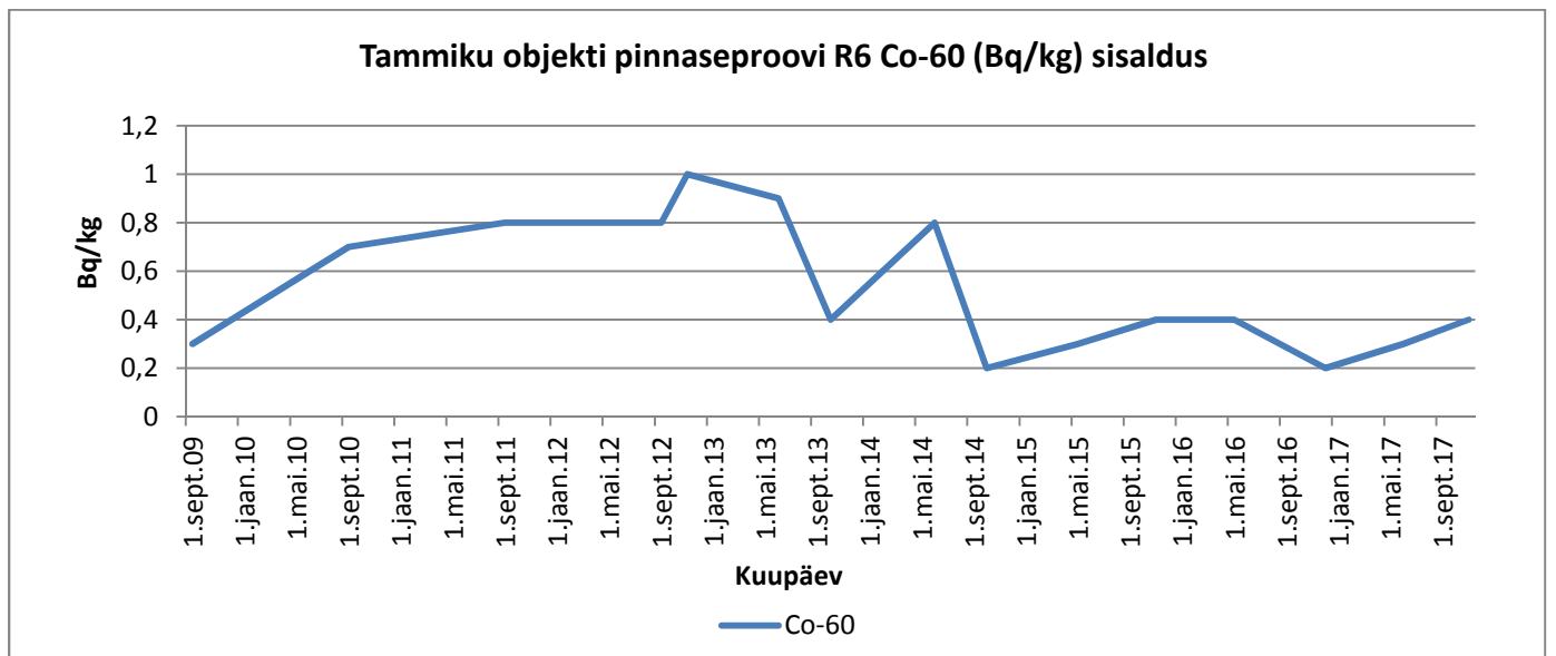
Graafik 33. Co-60
