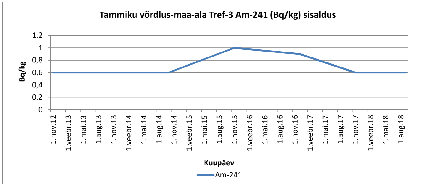
Graafik 81. Am-241
