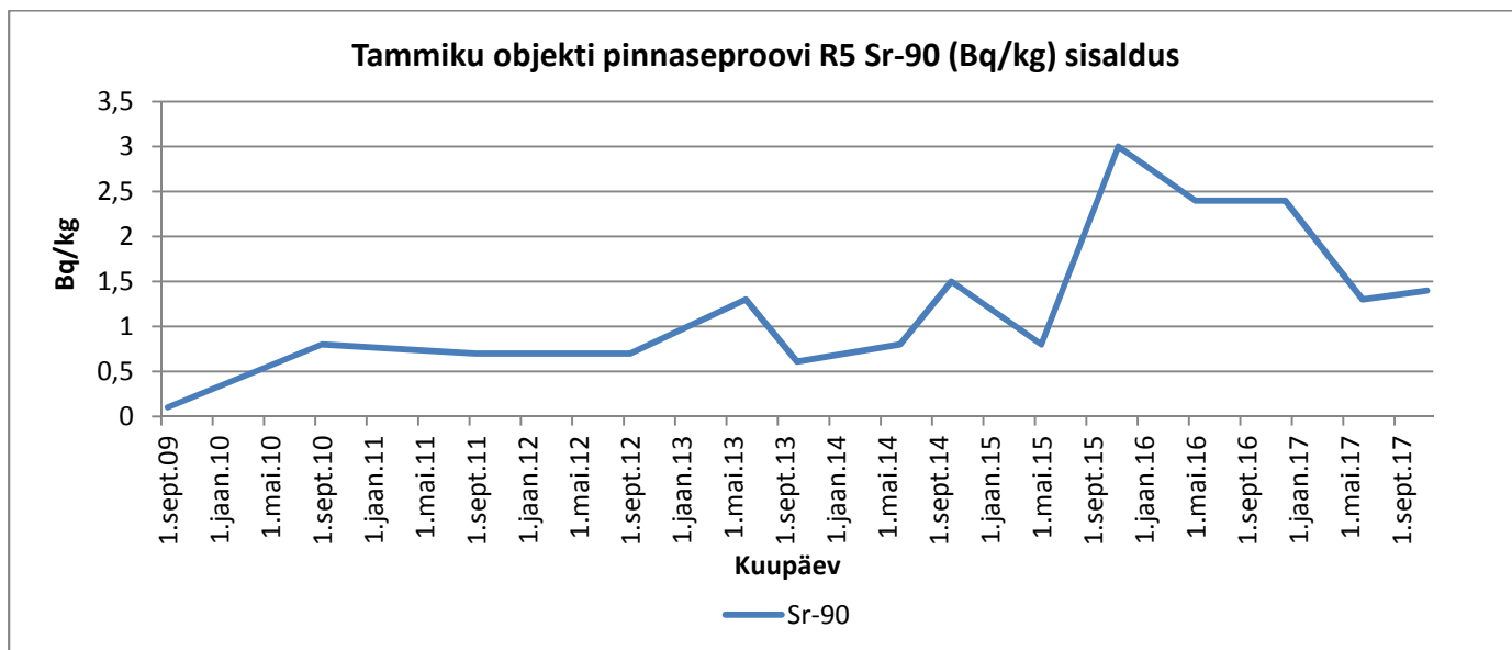
Graafik 27. Sr-90
