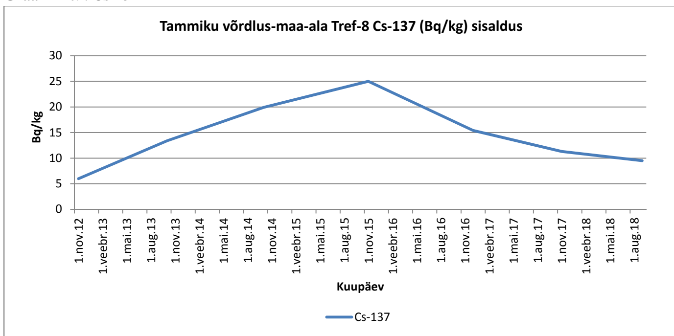
Graafik 109. Cs-137
