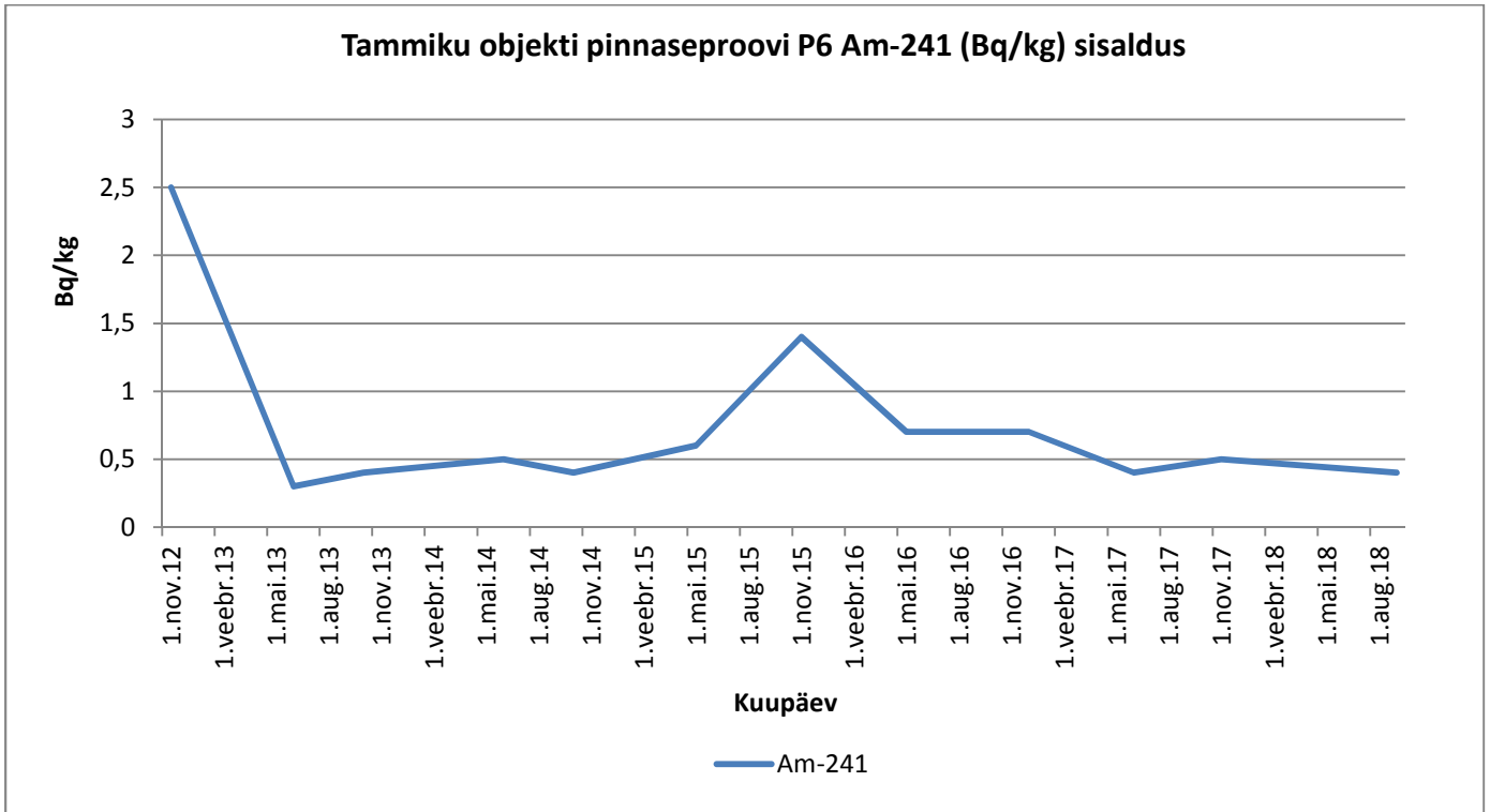
Graafik 55. Am-241
