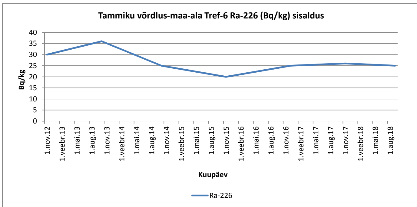
Graafik 100. Ra-226
