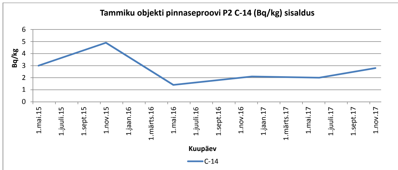
Graafik 45. C-14
