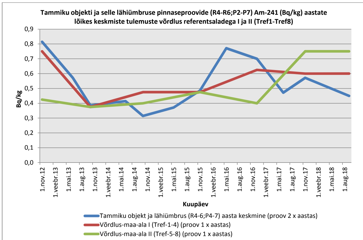
Graafik 120. Am-241
