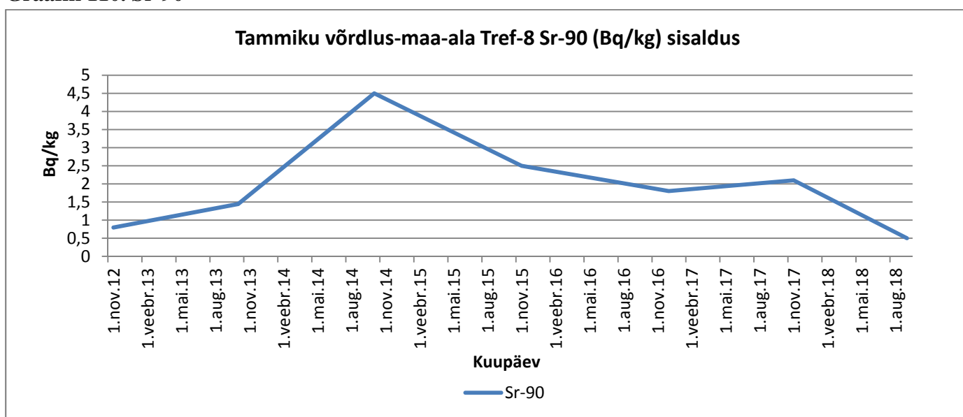
Graafik 110. Sr-90
