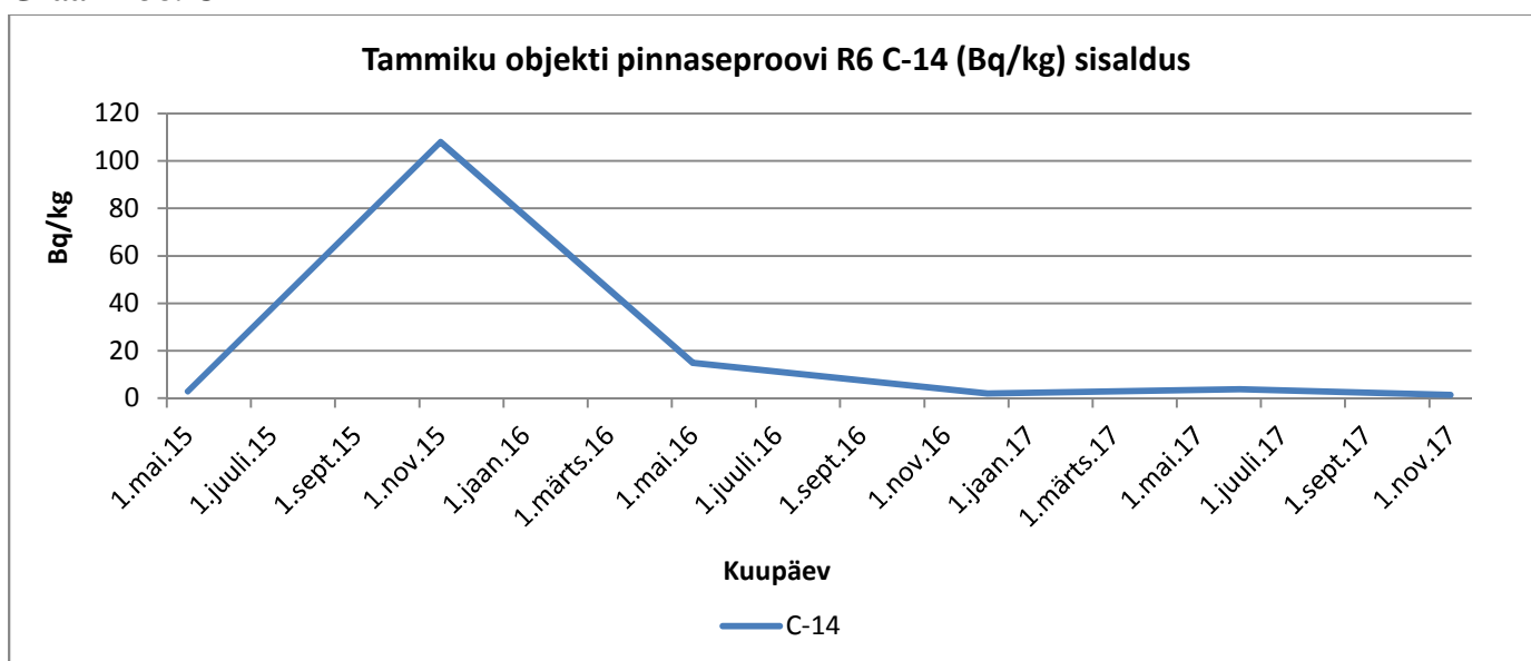
Graafik 38. C-14
