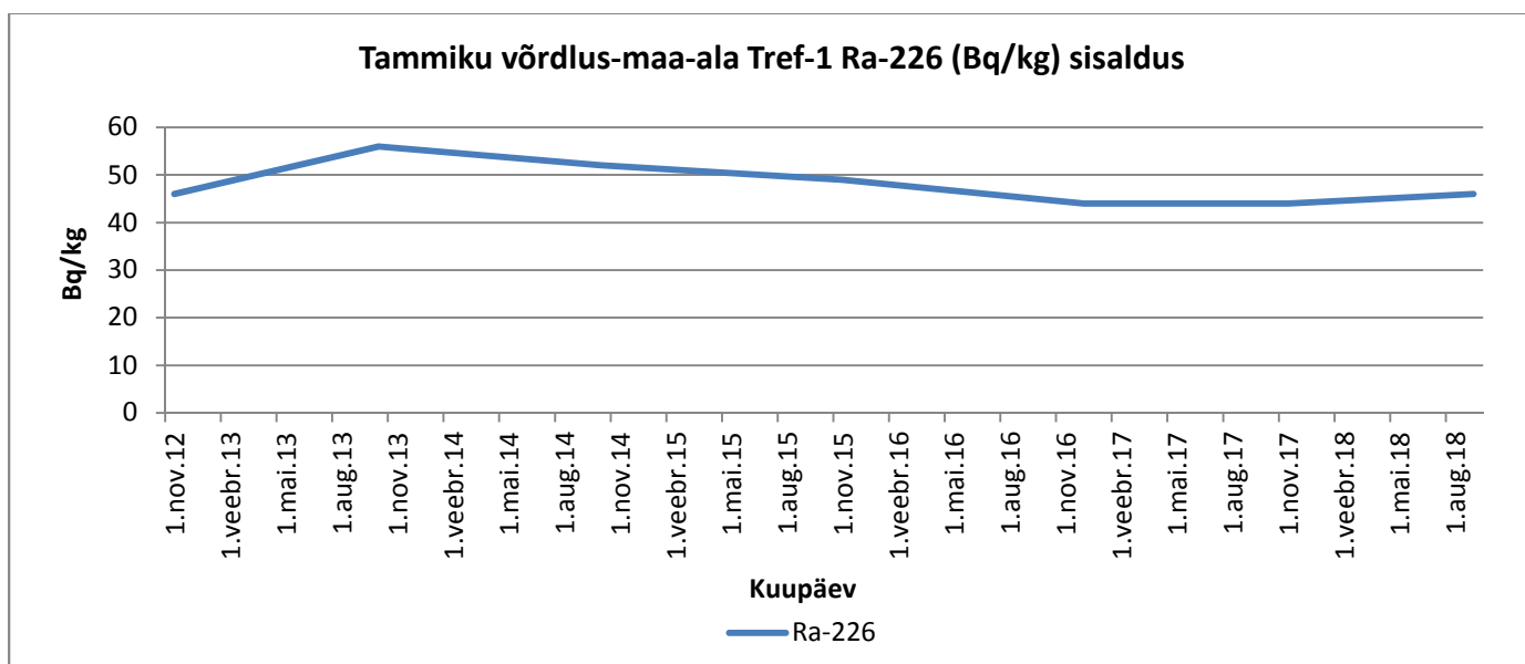
Graafik 70. Ra-226
